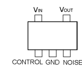
TAR5S30 (Q1063)
