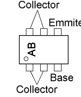
CPH6102 (AB) (Q1061, 1078)
