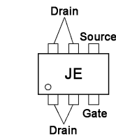
MCH6305 (JE) (Q1073)
