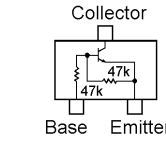
DTC144EM (26) (Q1031, 1039)
