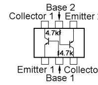
EMB3 (B3) (Q1029)
